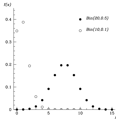
Figura 4.3: Ejemplos de funciones de distribución de probabilidad binomiales Bin(n, p) . Se han considerado dos modelos: Bin(20, 0.5) y Bin(10, 0.1)
