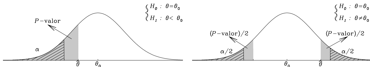
Figura 9.4: Esquema del cálculo del P -valor para un contraste bilateral (a la derecha) y para un contraste unilaterial izquierdo (a la izquierda).
